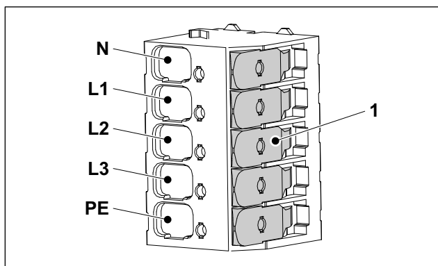
Abb. 5 Anschlussklemmen der Spannungsversorgung
